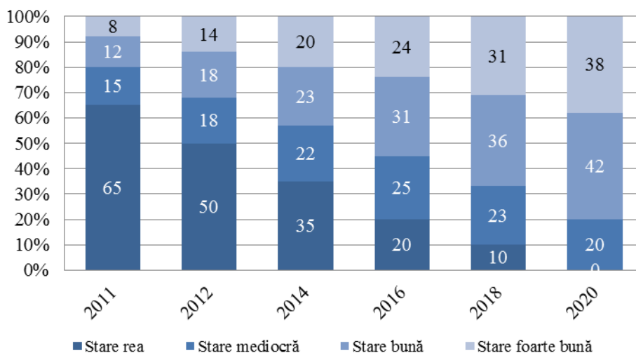
Figura 8. Prognosticul evoluției stării drumurilor naționale în perioada anilor 2011-2020
